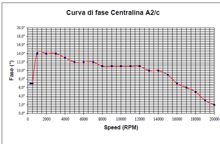
Curva di fase dell'accensione SELETTTRA A2/c Statore 2 Poli Ø 58.
