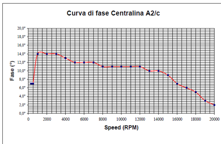
Curva di fase dell'accensione SELETTTRA A2/c Statore 2 Poli O 58.
