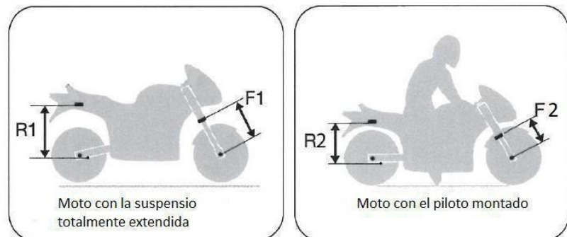
Ilustración 7: Reglaje y ajuste de chasis
