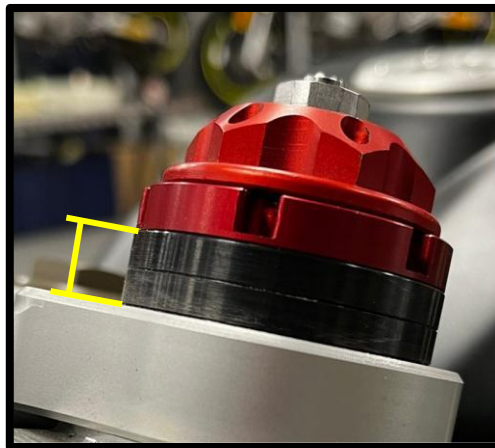
Ilustración 5: Ajuste de altura de barras
